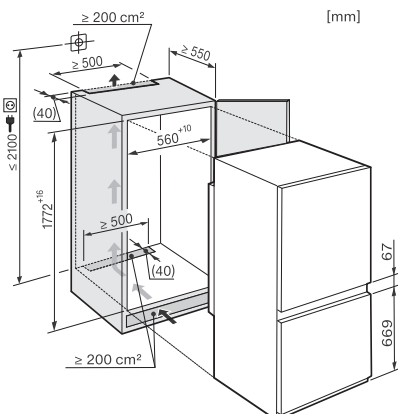
Zabudovateľná chladnička s mrazničkou KFN 7733 F
