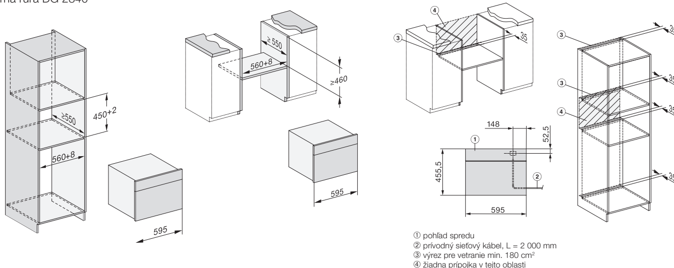
Parná rúra DG 2840
