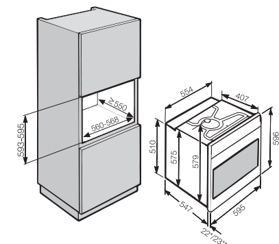
Zabudovateľná rúra na pečenie H 2860-2 B/BP, H 7262 B/BP
